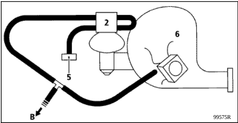
SCHEMA FONCTIONNEL DU CIRCUIT PNEUMATIQUE
