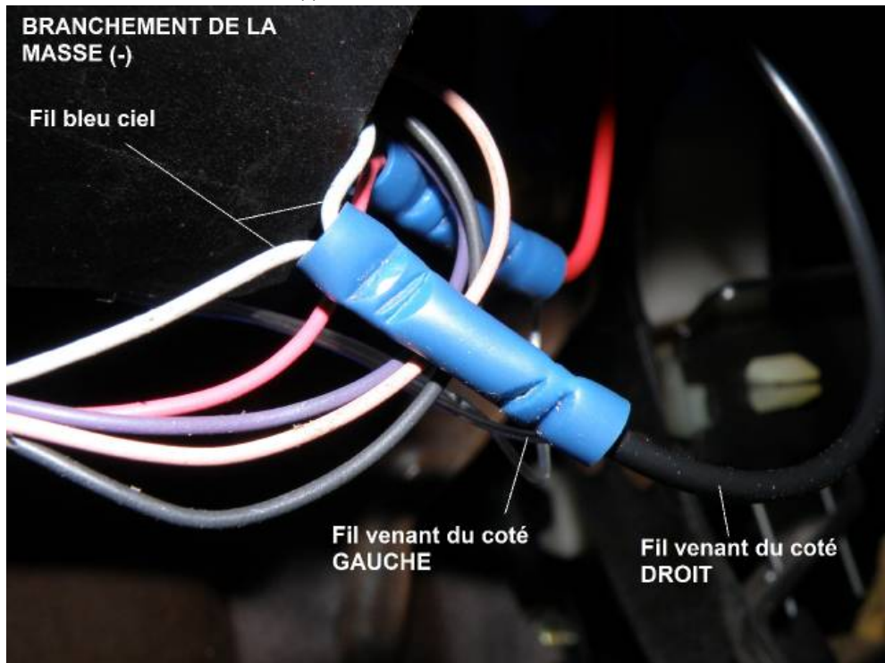
Branchement de la masse (-)
