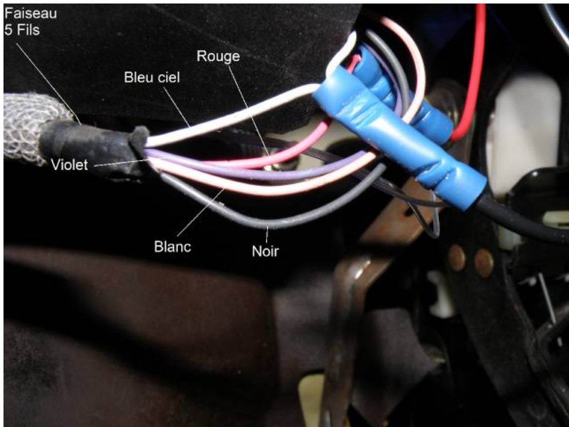
Branchement de la masse (-)
